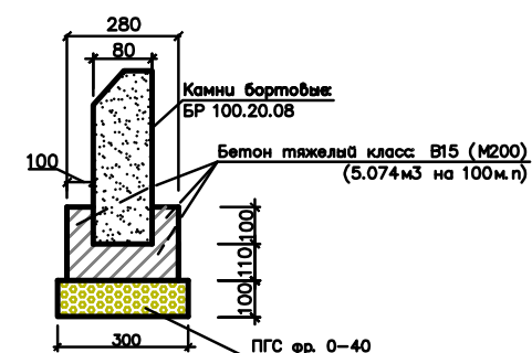
Узел бортового камня БР 100.20.8
