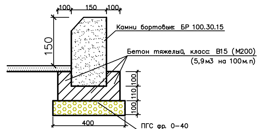
Узел бортового камня БР 100.30.15
