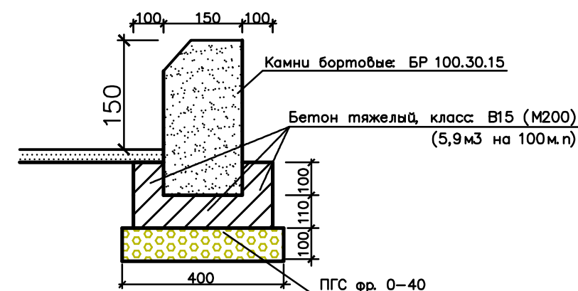
Узел бортового камня БР 100.30.15
