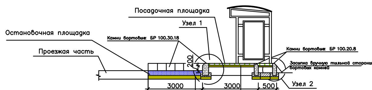
Разрез А-А
