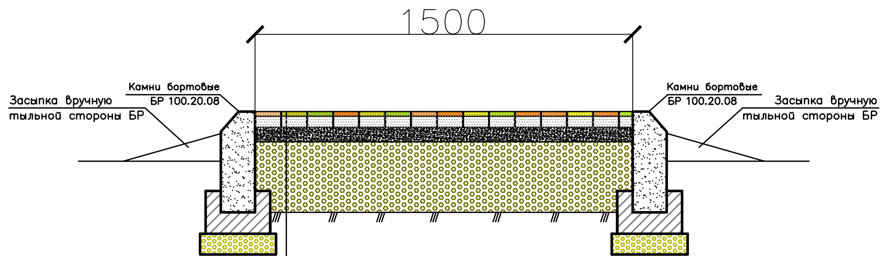
Конструктив тротуара Разрез 2-2
