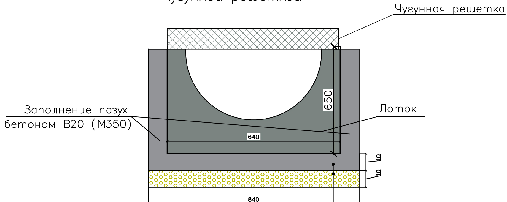
Узел водоотводного ж/б лотка с чугунной решеткой
